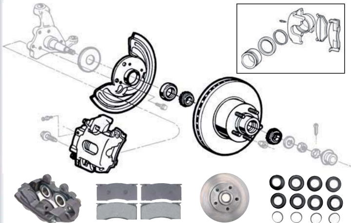
FRC4176 Disc Brake Caliper
